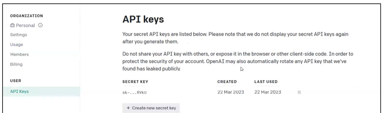
Fig. 3: API Keys
